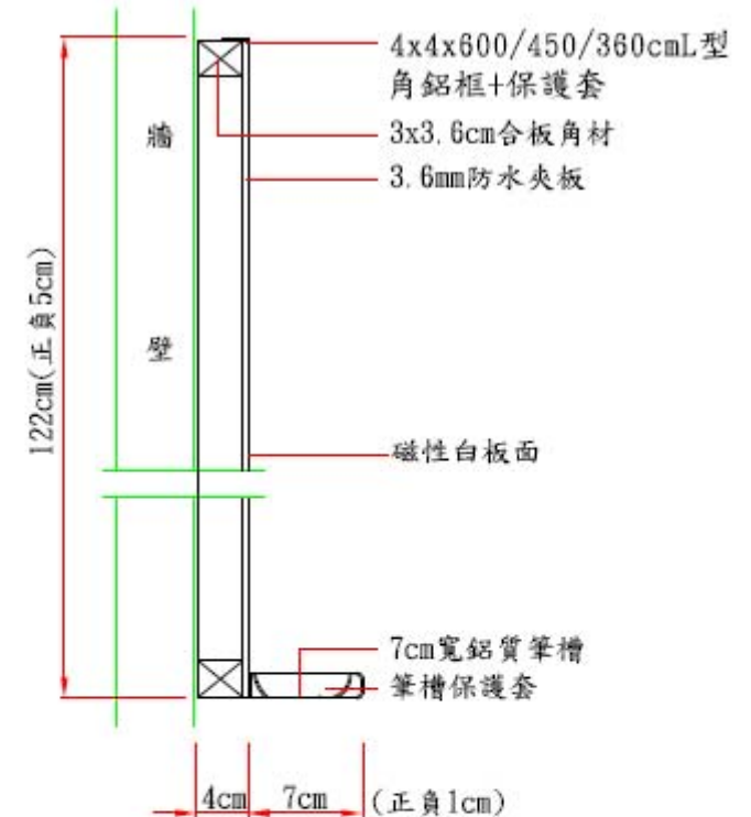
鋁框平面磁性白板側視圖
