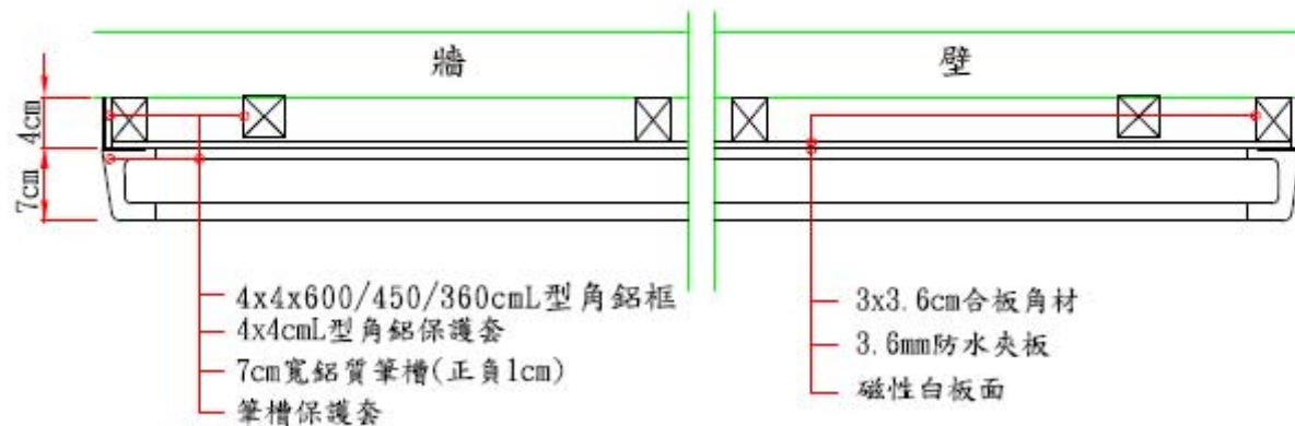
鋁框平面磁性白板上視圖
