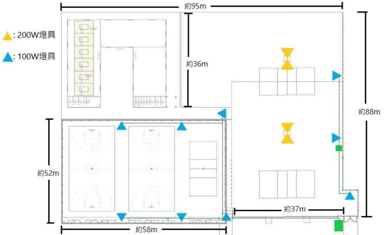
校本部 綜合球場 安裝位置圖
